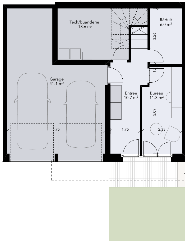
VILLA D1 - NIVEAU 0 (Accès)
