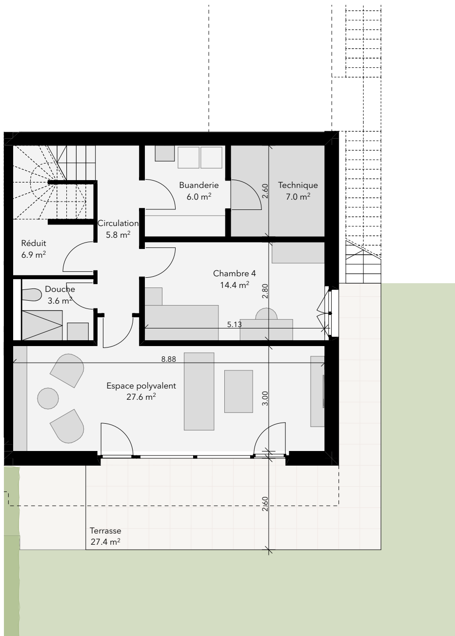
VILLA A2 - NIVEAU 0 (Jardin)
