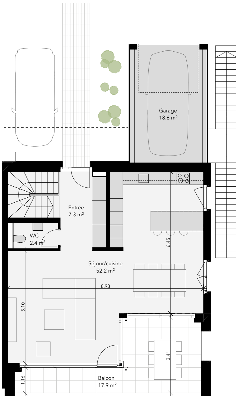
VILLA A2 - NIVEAU 2 (Accès)
