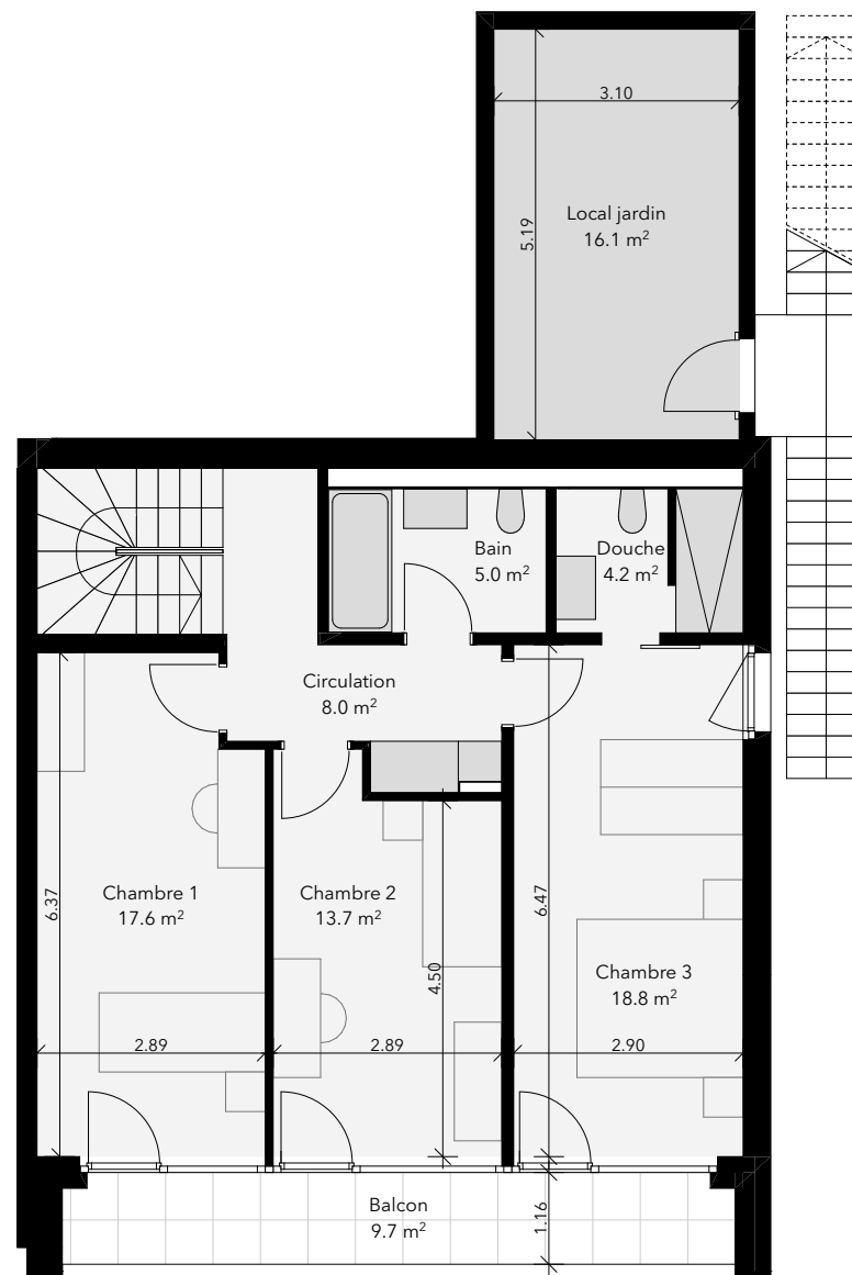
VILLA A2 - NIVEAU 1
